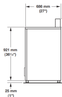
Vista posterior
