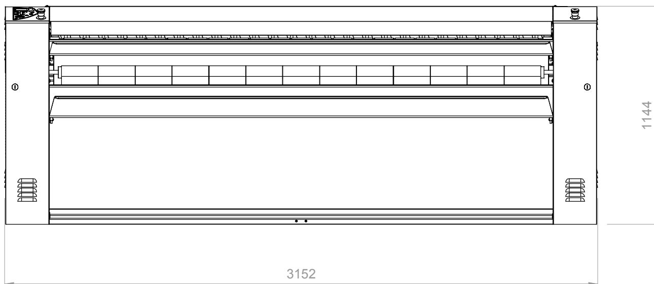
FRONTAL
